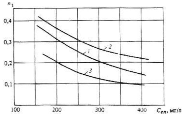
Черт. 2. Зависимость показателя степени n_1 от исходной концентрации взвешенных веществ в городских сточных водах при эффeкте отстаивания
